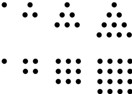
Треугольные и квадратные числа
