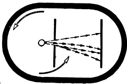
Рис. 12. Устройство прибора для определения скоростей молекул.
