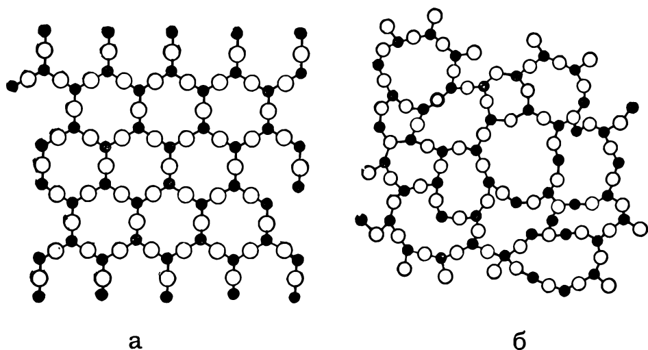
Рис. 58: а — строение кристалла, б — строение аморфного стекла.
