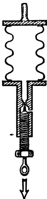
Рис. 26. Прибор для определения сопротивления жидкости разрыву.
