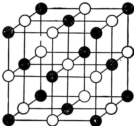
Рис. 45. Кристаллическая решетка поваренной соли.
