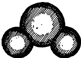
Рис. 6. Молекула воды.
