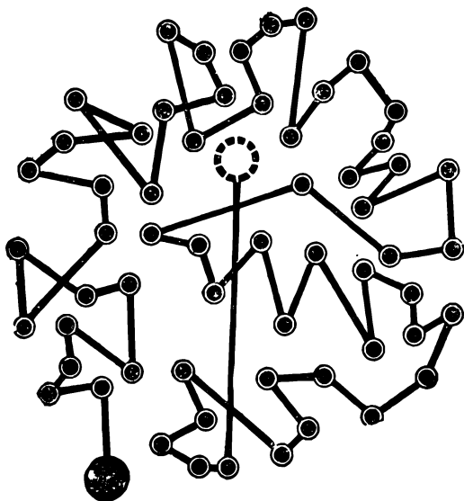
Рис. 10. Схема броуновского движения.
