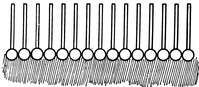
Рис. 37. Строение поверхностного слоя водного раствора мыла.
