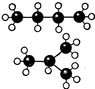
Рис. 7. Две молекулы, различающиеся расположением атомов.
