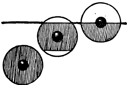
Рис. 24. Молекулы в поверхностном слое жидкости.
