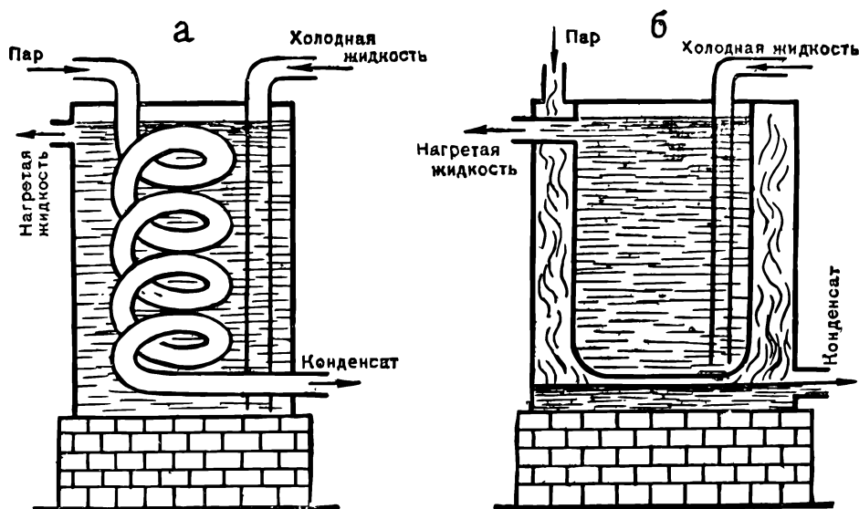
Рис. 40. Паровые нагреватели: а — змеевик, б — „паровая рубашка“.
