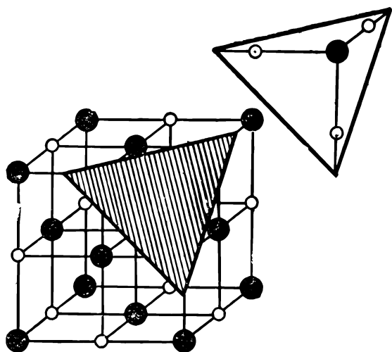
Рис. 52. Диагональные плоскости в кристалле поваренной соли.
