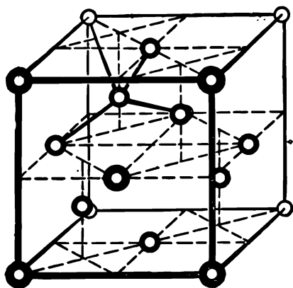
Рис. 47. Кристаллическая решетка алмаза.
