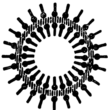
Рис. 38. Поверхностные слои в мыльном пузыре.
