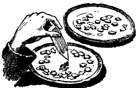
Рис. 36. Разбегание бумажек по поверхности воды.
