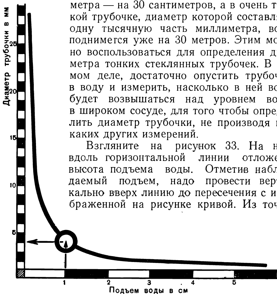
Рис. 33. График для определения диаметра капилляра.
