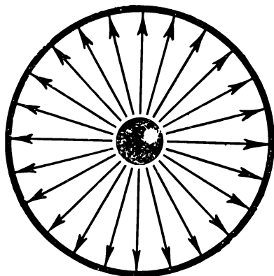
Рис. 23. Сфера молекулярного действия.
