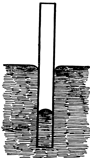
Рис. 32. Несмачивающая жидкость в капилляре.
