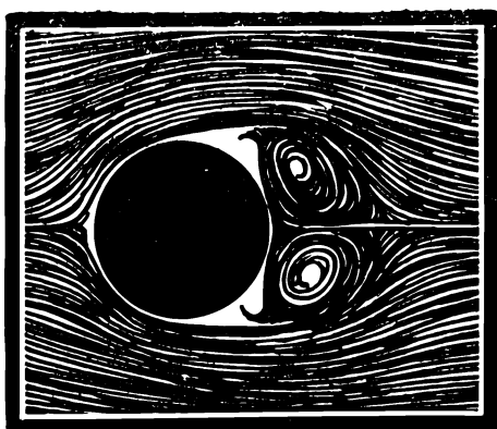
Рис. 42. Вихри в жидкости.
