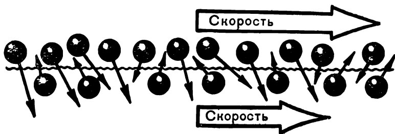
Рис. 43. Возникновение внутреннего трения в газе.
