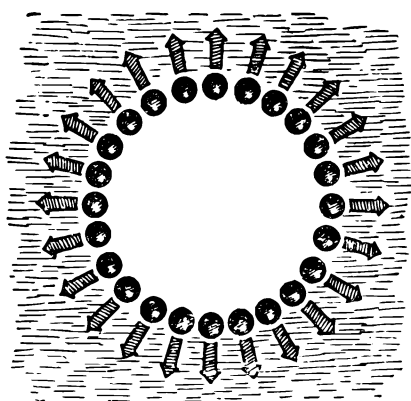
Рис. 25. Молекулярное давление всегда направлено в глубину жидкости и уравновешивается взаимным отталкиванием частиц.
