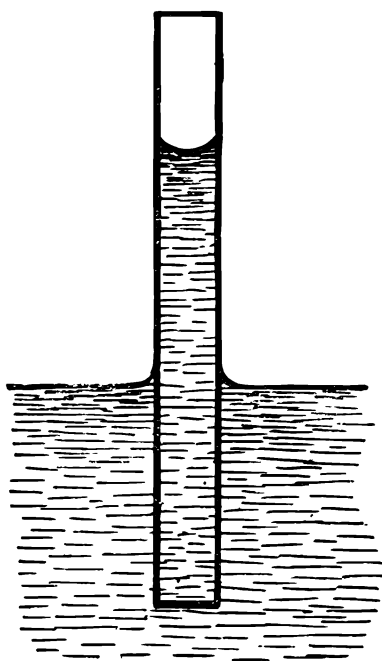
Рис. 31. Смачивающая жидкость в капилляре.
