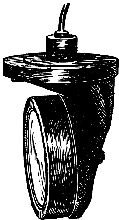
Рис. 57. Пьезоэлектрический излучатель ультразвука.
