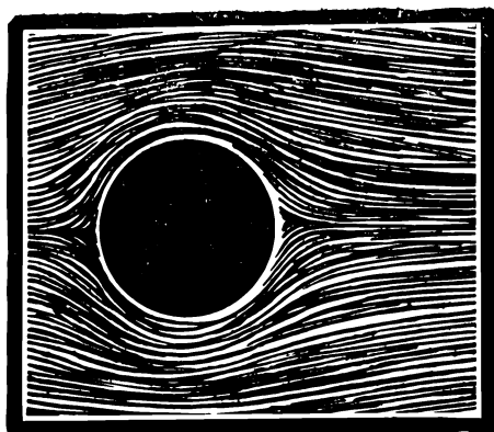
Рис. 41. Слоистое течение жидкости.
