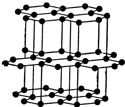
Рис. 46. Кристаллическая решетка графита.
